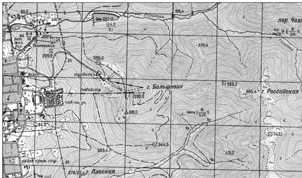
Ил. 1. Фрагмент топографической карты восточных окрестностей Южно-Сахалинска.
